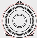
Lochkreis: 121mm
